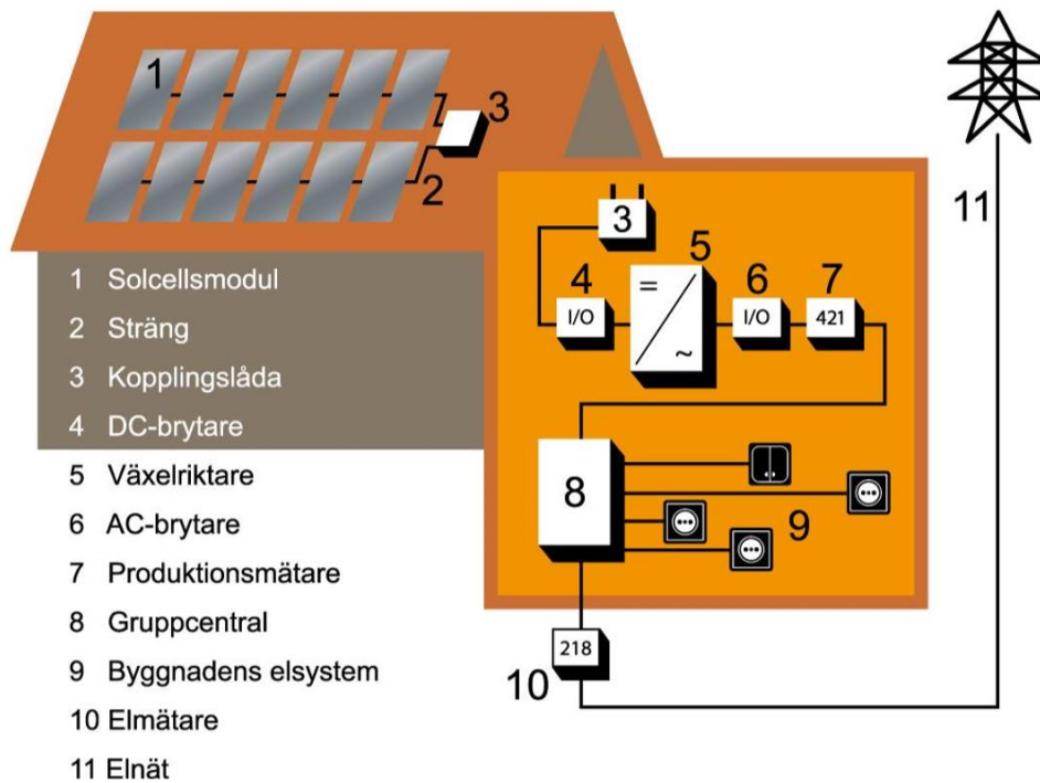
Figur 11: Ett solcellssystem
