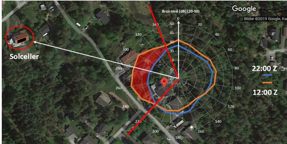
Figur 21: Störnivån varierar när anmälarens antenn roteras ett varv vid två olika tillfällen.
