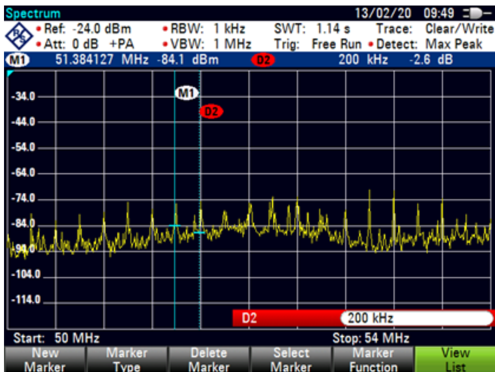
Figur 26: Störande signaler.
